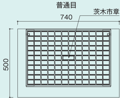
上部ブロック平面図
