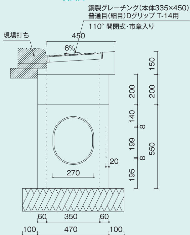
側面図
