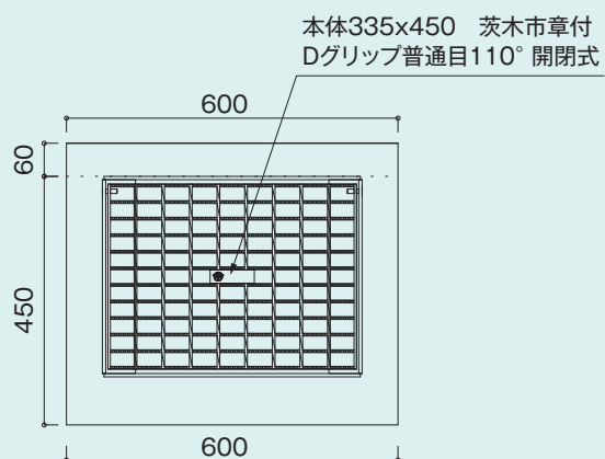
上部ブロック平面図
